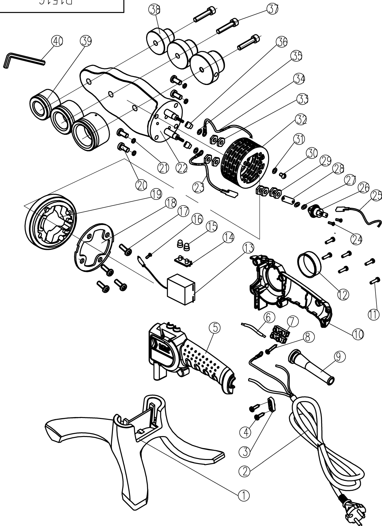
爆炸图
